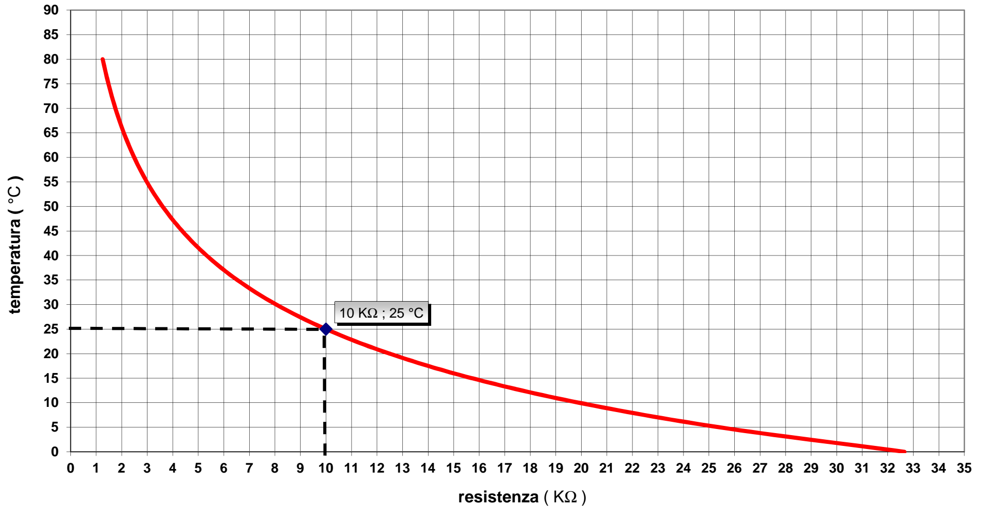
COD 1.023405 grafico resistenza-temperatura sonda NTC ingresso sanitario per eolo superior kw
