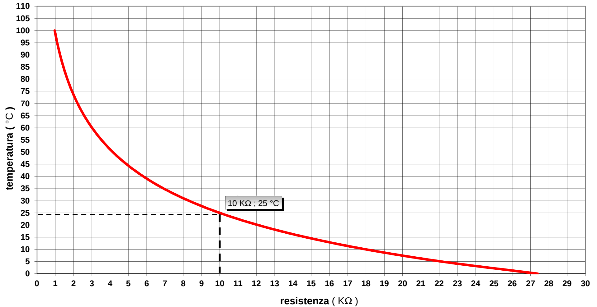
COD 1.024296 grafico resistenza-temperatura sonda NTC fumi per modulo Isothermic
