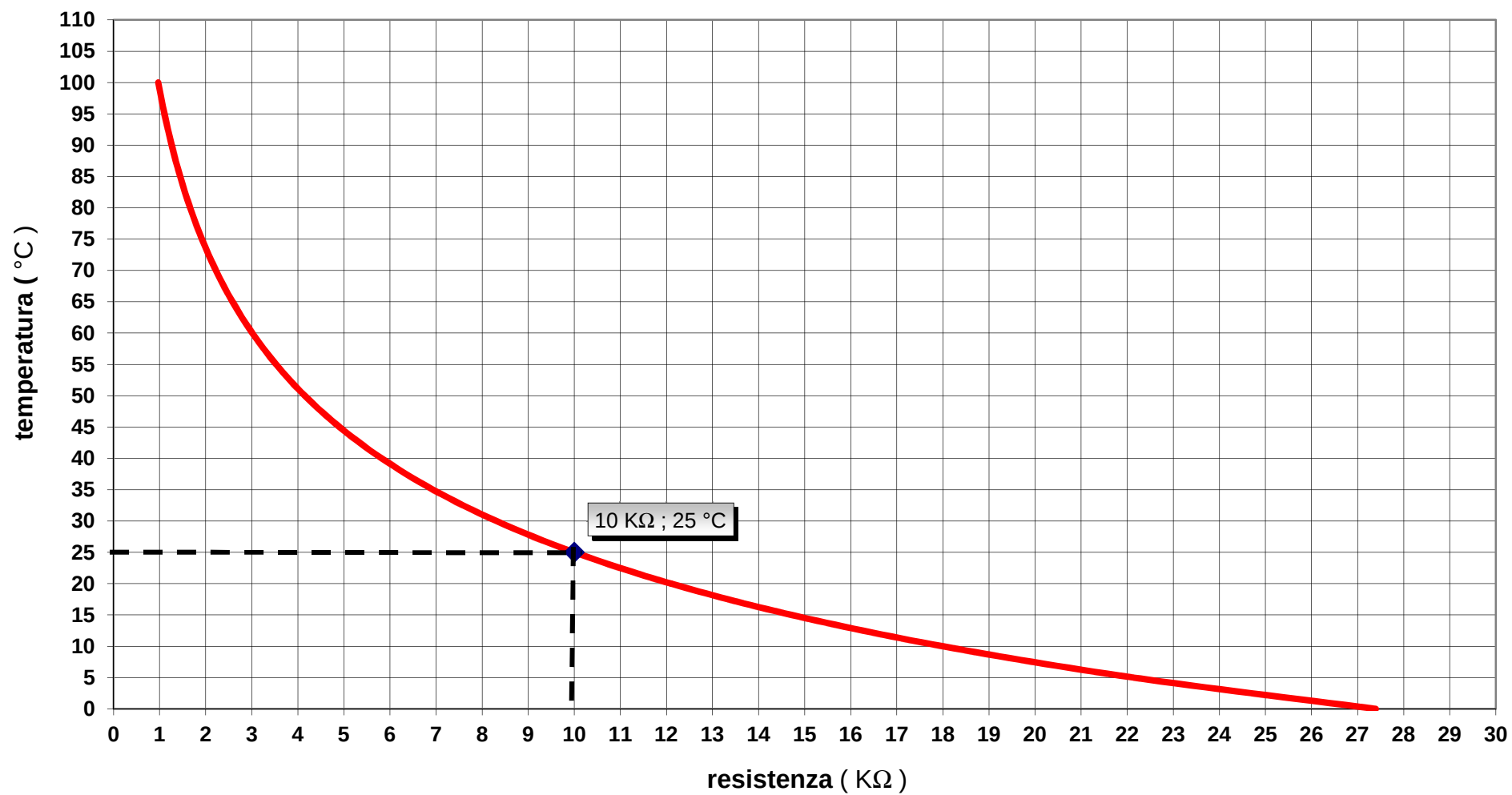
COD 1.028266 grafico resistenza-temperatura sonda NTC rossa Thermodisc
