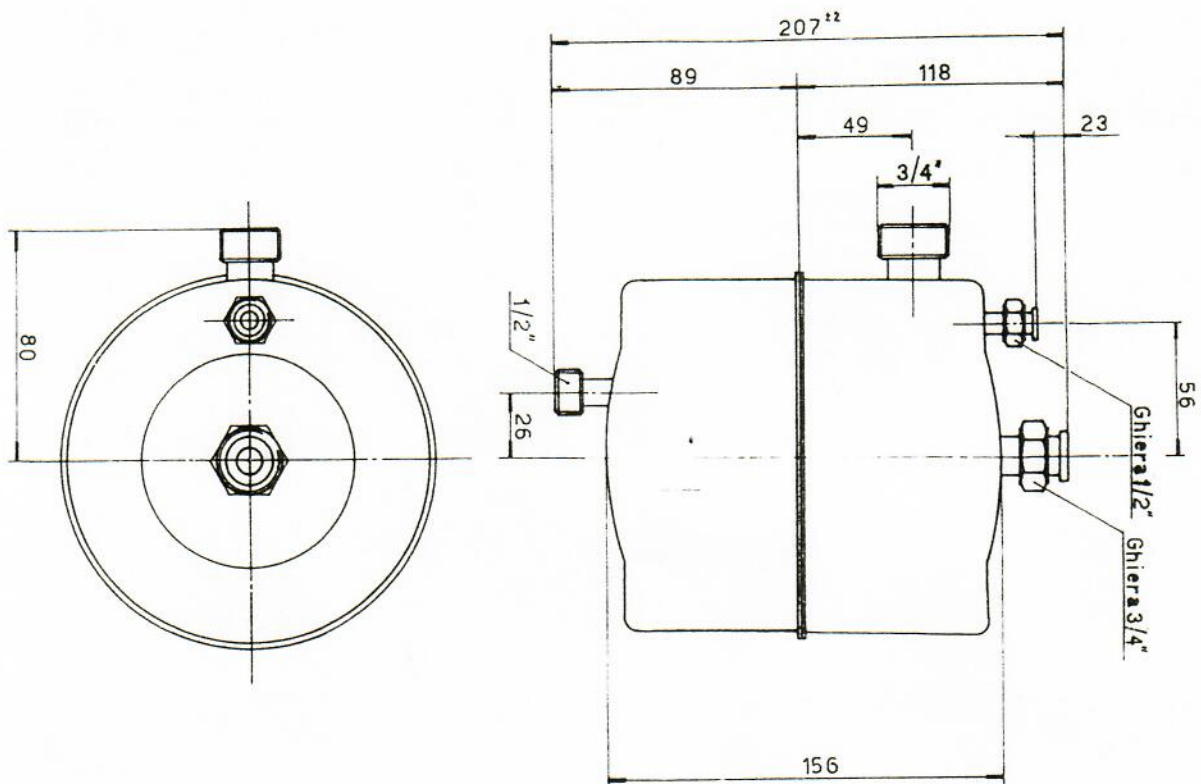
MOD. 1/8 PER CALDAIA NEW FAR MERLONI
