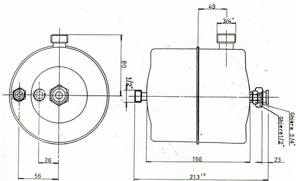
MOD. 27/8 PER CALDAIA EUROTERM FINTERM
