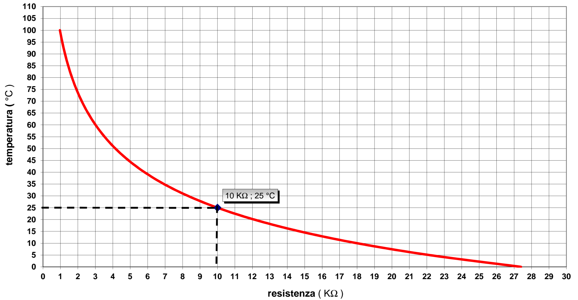
COD 1.033683 grafico resistenza-temperatura sonda NTC boiler per abbinamento caldaie inf. 35 kw
