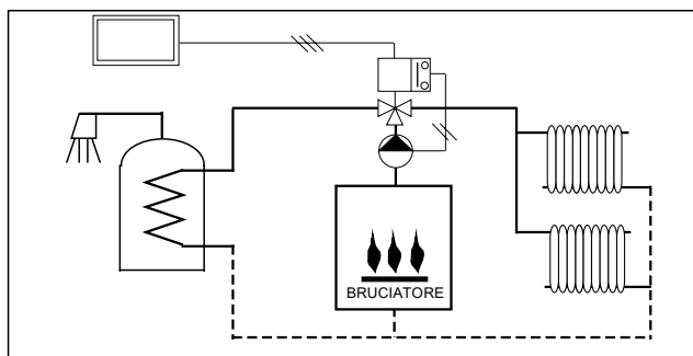
VC4613M.. Valvola a 3 vie con comando SPST . Produzione Acqua Calda Sanitaria
